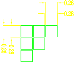
DOT DETAIL SCALE:20:1
